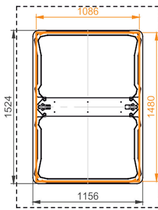
Côtes au sol de l'étage
