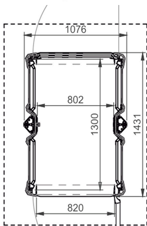
Côtes gaine et porte
